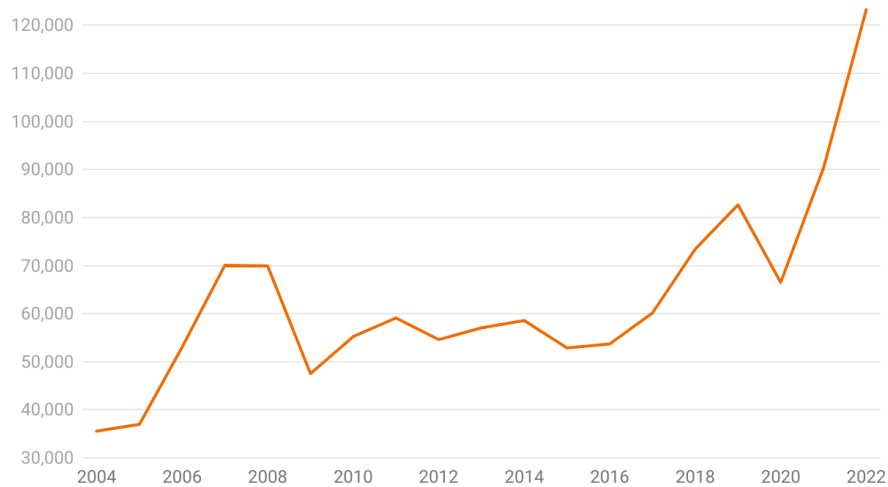
Figura 4: posti vacanti
